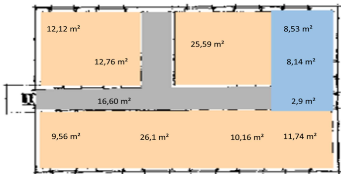
GRUNDRISS ERDGESCHOSS
